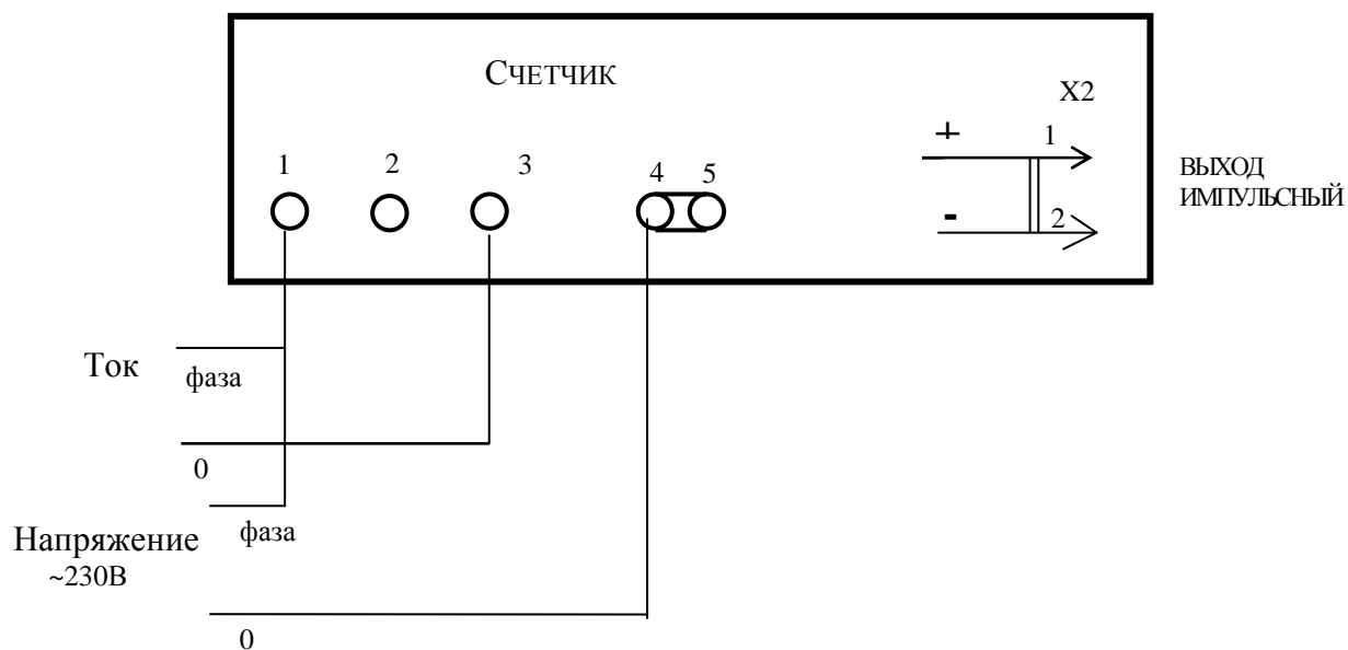
Рисунок 1 – Схема подключения счетчиков при поверке СЭО-1.09.302, СЭО-1.09.302А, СЭО-1.09.302/1, СЭО-1.09.302А/1, СЭО-1.09.502, СЭО-1.09.502А, СЭО-1.09.502/1, СЭО-1.09.502А/1
