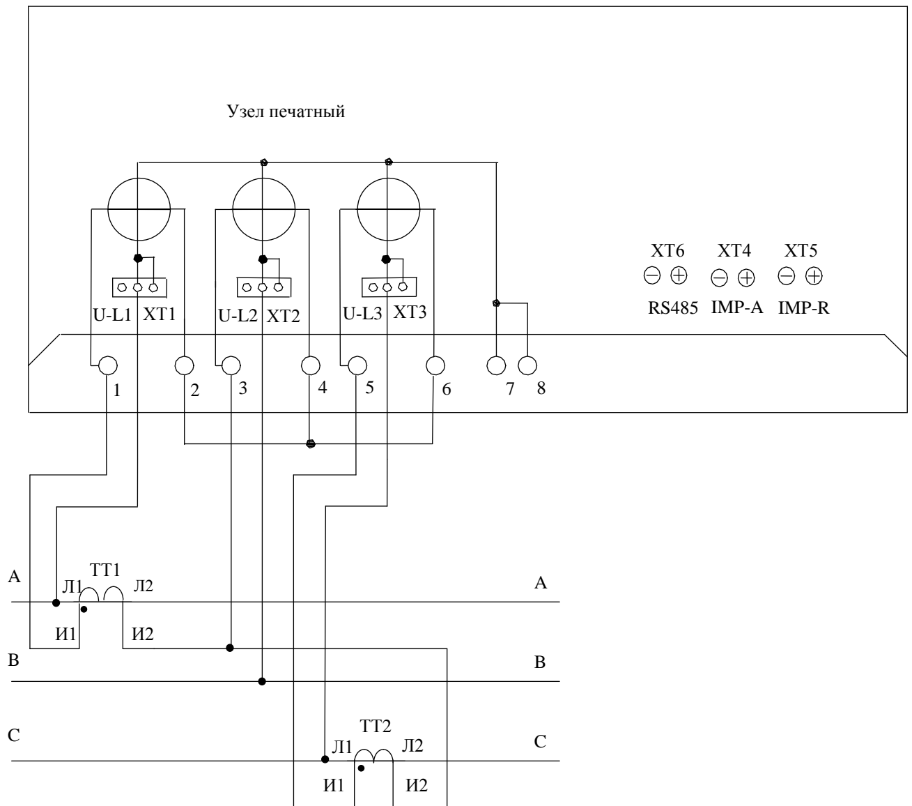
Рисунок Б.4 – Схема подключения счётчика к трёхфазной трёхпроводной сети с помощью двух трансформаторов тока
