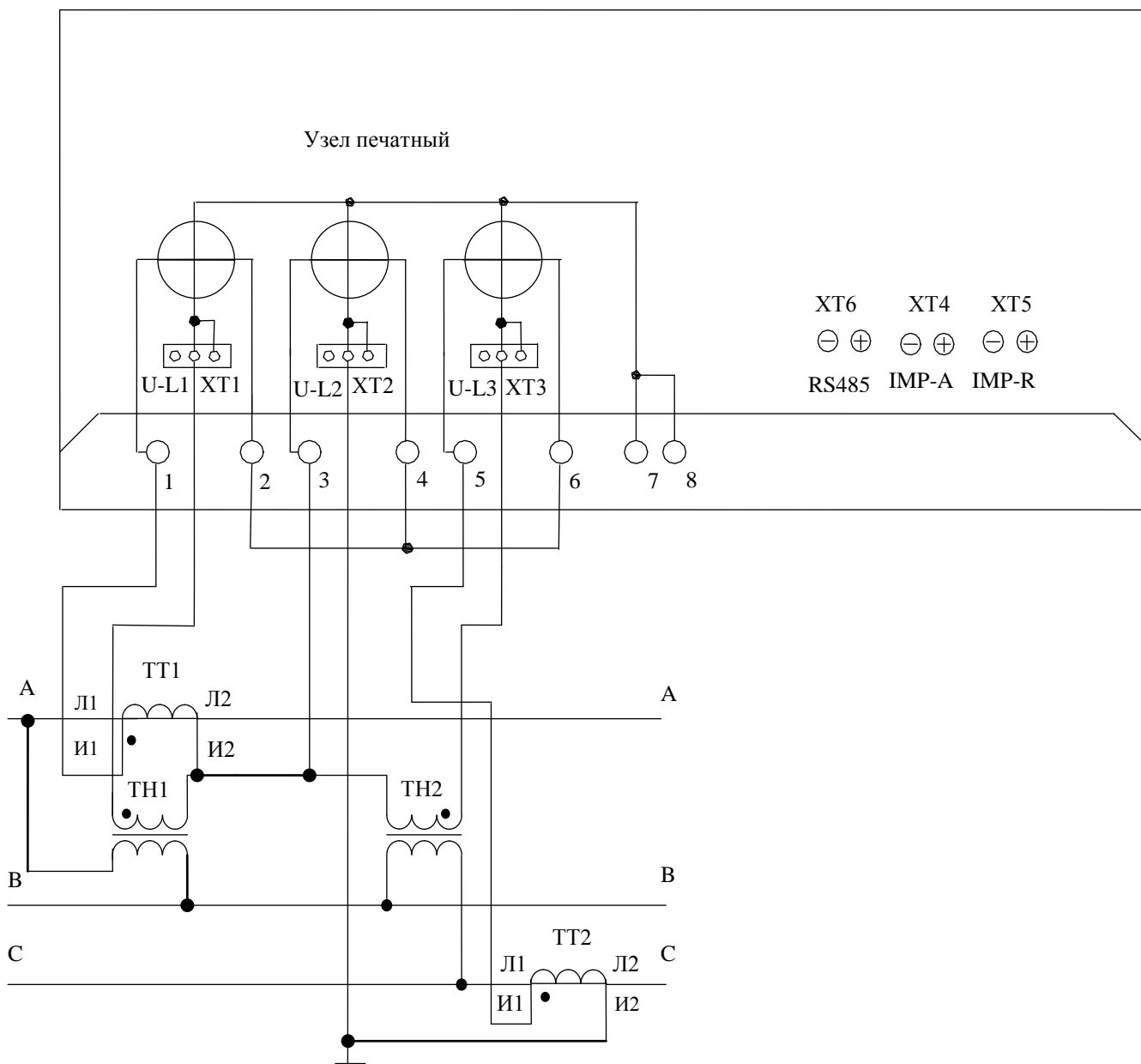
Рисунок Б.6 - Схема подключения счётчика к трёхфазной трёхпроводной сети с помощью двух трансформаторов напряжения и двух трансформаторов тока
