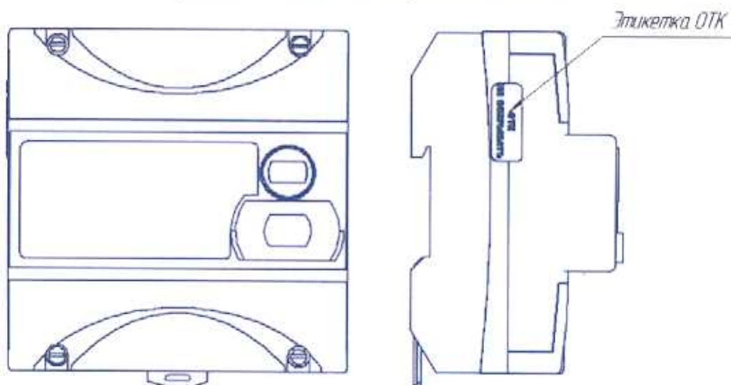
Рисунок 2 – Схема пломбирования счётчика
