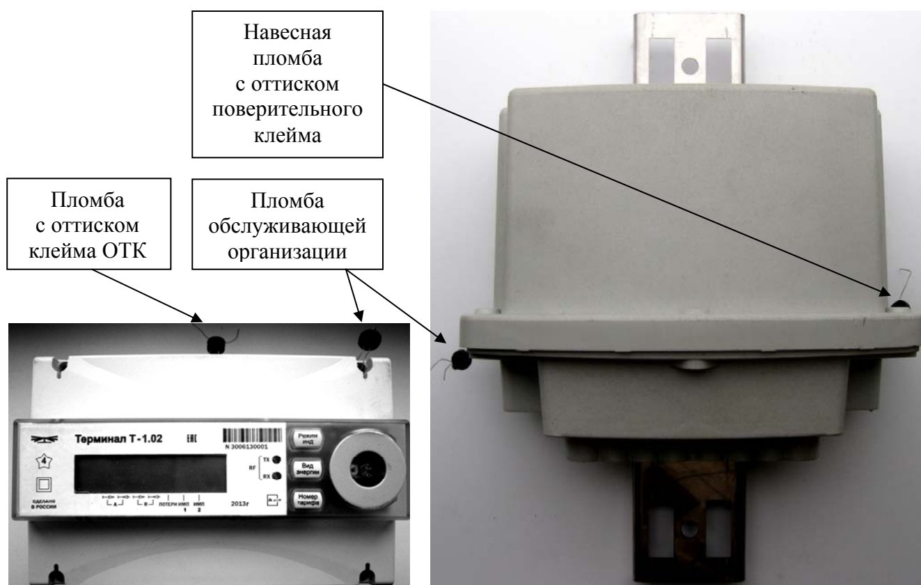
Рисунок 1 – Внешний вид счётчика наружной установки и терминала Т-1.02
