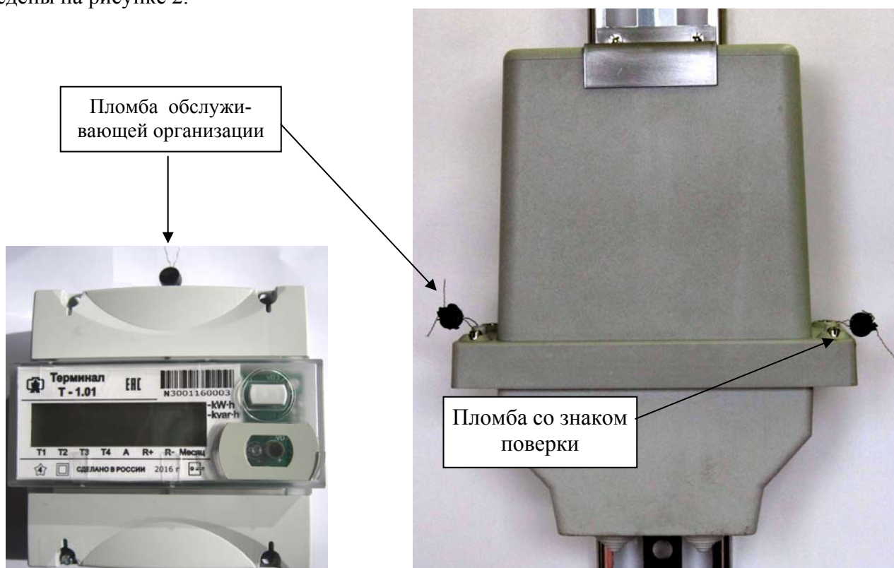
Рисунок 2 – Внешний вид счетчиков наружной установки и схема пломбирования
