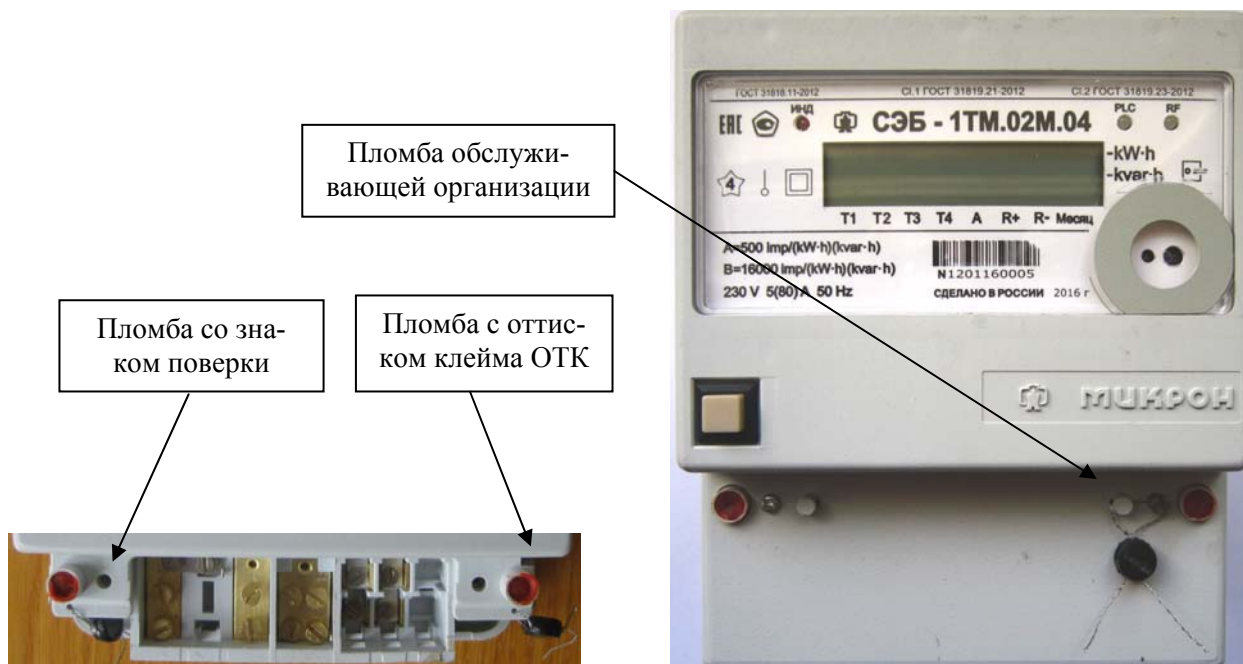
Рисунок 1 – Внешний вид счетчиков, предназначенных для установки внутри помещения, и схема пломбирования
