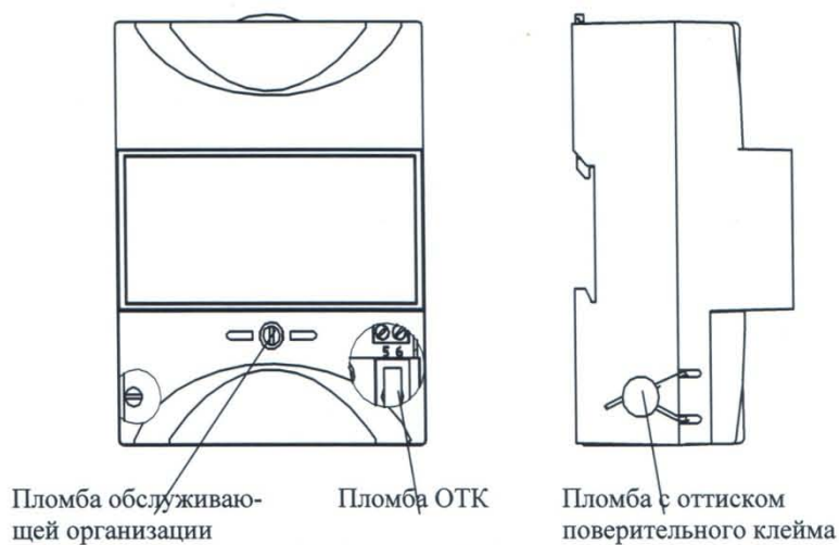
Рисунок 2 – Схема опломбирования счетчиков
