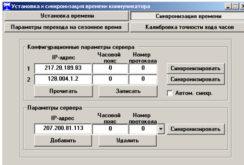
Рисунок 8 - Форма «Установка и синхронизация времени коммуникатора», вкладка «Синхронизация времени»
