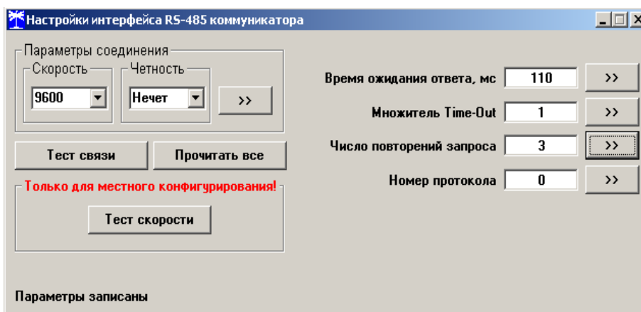
Рисунок 4 - Форма «Настройки интерфейса RS-485 коммуникатора»
