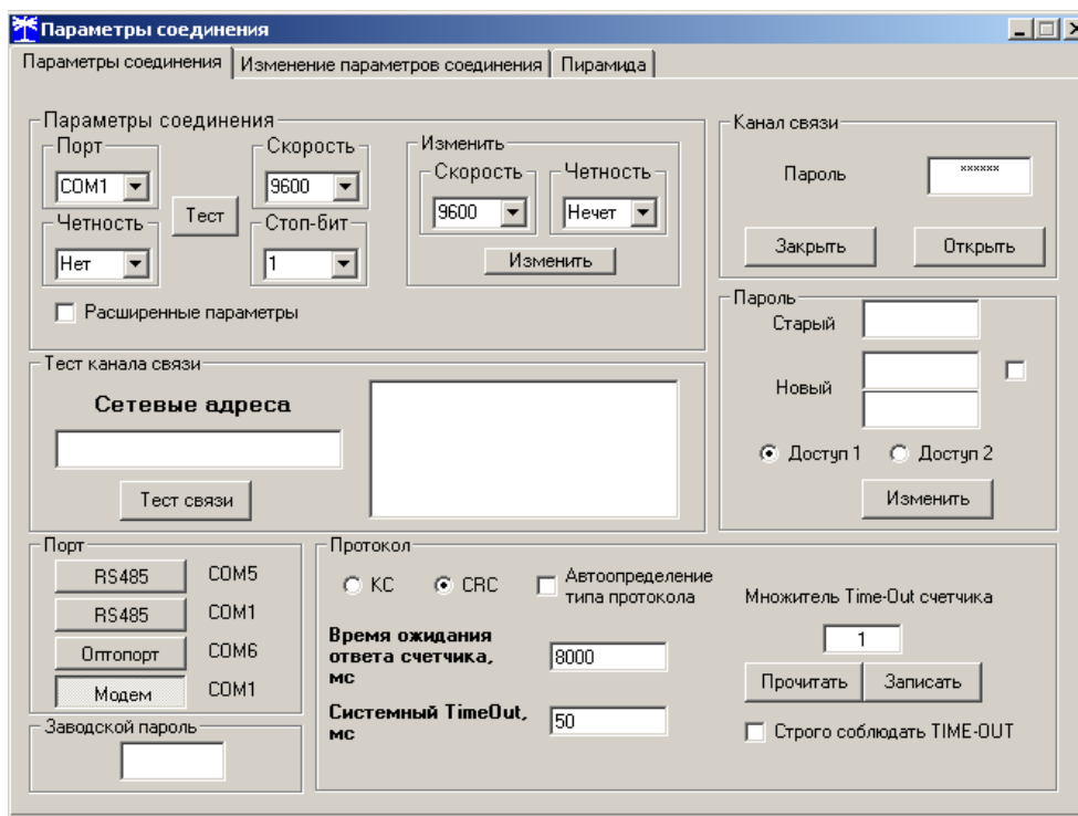
Рисунок 12 – Параметры соединения с GSM-модемом
